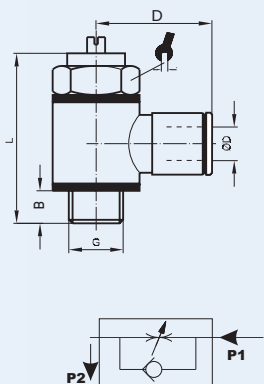
用于阀门平行的流量调节器
