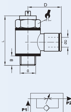
用于气缸平行的流量调节器
