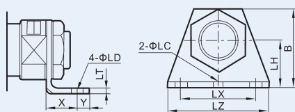
脚座 Foot Base
