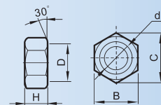
杆端螺母 Rod Nut
