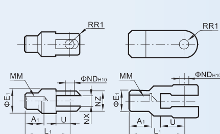
Y型肘节接头 Y Fitting
