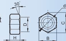
安装螺母 Fixing Nut
