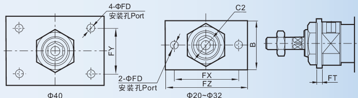
法兰 Flange
