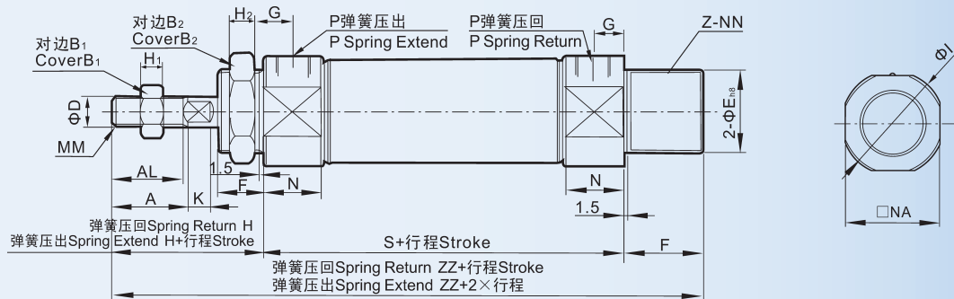
基本型 Basic Type
