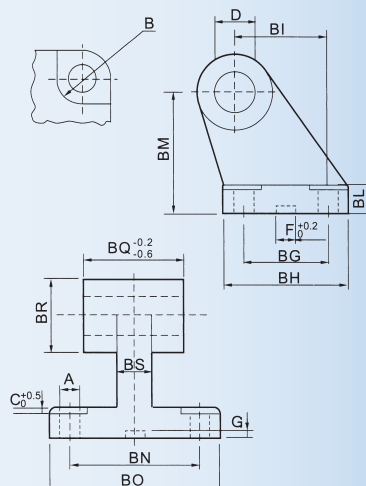
SDB 后盖固定型 (斜耳环) Back Cover Fixed Type
