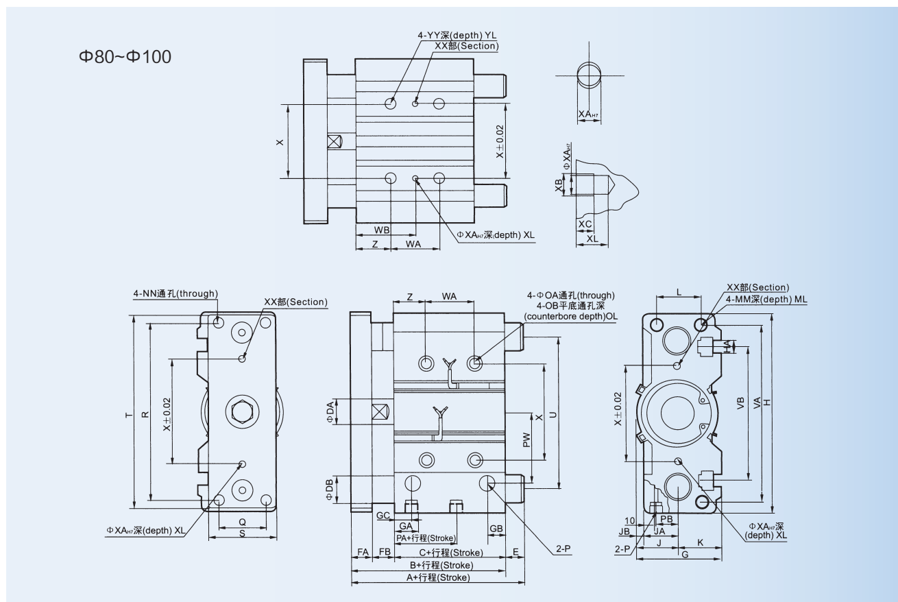
MGPM, MGPL尺寸表 (Φ80~Φ100)
